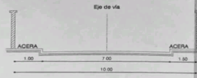
CORTE TIPO VIA DE 10.00 m
