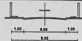
CORTE TRANSVERSAL CALLE PUBLICA
