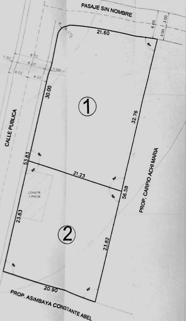
PLANO PLANIMETRICO
