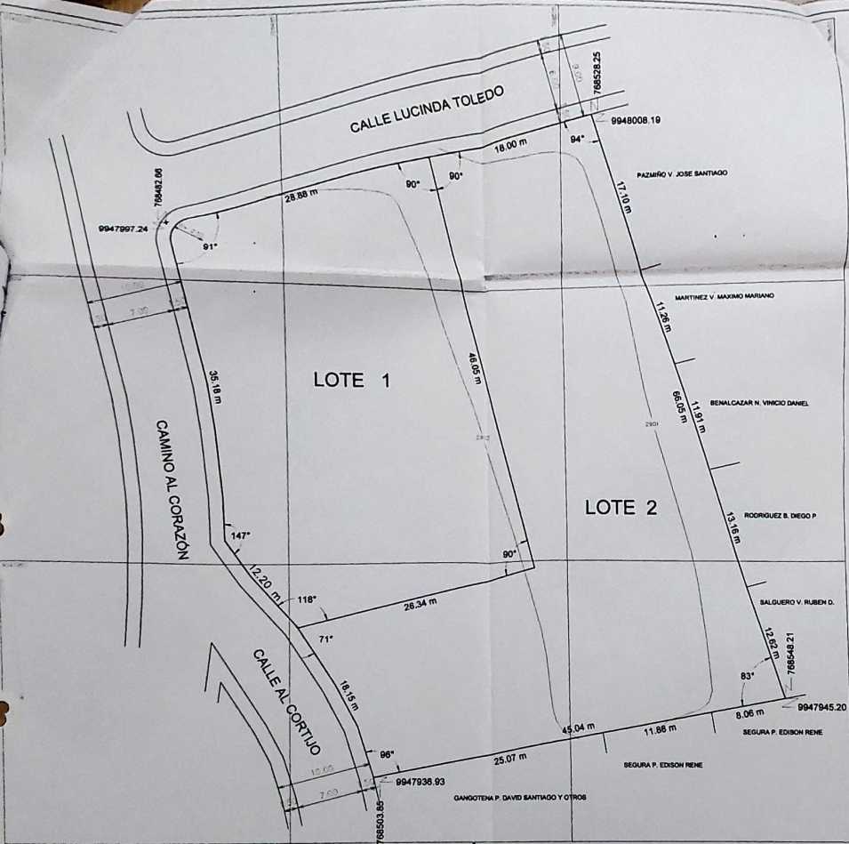
PLANO DE FRACCIONAMIENTO ESC. 1/250
