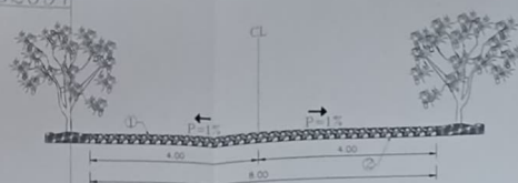
CORTE TÍPICO DE LA VÍA EXISTENTE ESCALA _____ 1:50
