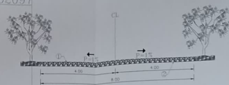
CORTE TÍPICO DE LA VÍA EXISTENTE ESCALA _____ 1:50
