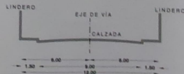
CORTE CALLE LOS EUCALIPTOS ESCALA 1:100
