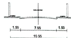
CORTE TRANSVERSAL CALLE SIN NOMBRE
